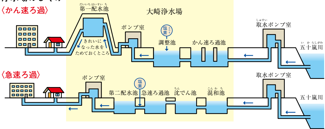
かん速ろ過池
